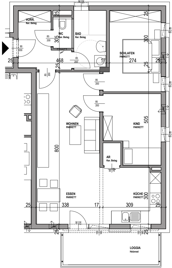
M=1:100 GRUNDRISS M=1:50 SIEHE FOLGEBLATT
